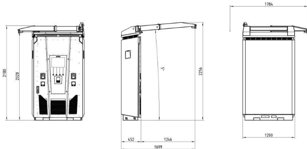
Mått eTower200
