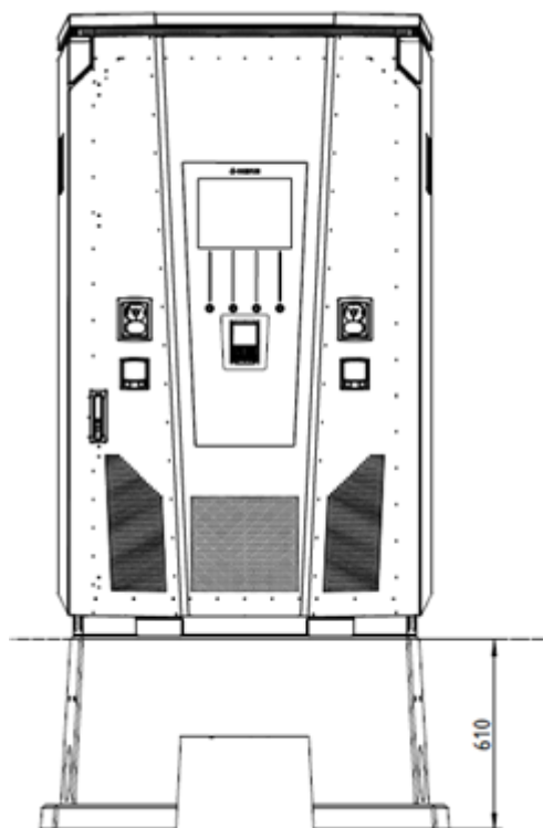
Mått betongsöcket
