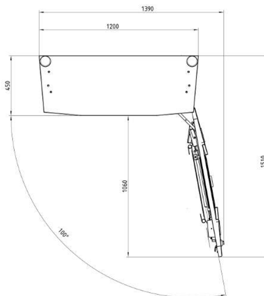
Dörrens öppningsvinkel
